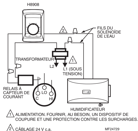
Fig. 10. Schéma de câblage avec humidistat H8908 (compris) et relais à détection de courant (non compris).*
