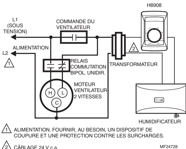
Fig. 9. Schéma de câblage avec humidistat H8908 (compris). Le transformateur est alimenté lorsque le ventilateur à deux vitesses est sous tension.*
